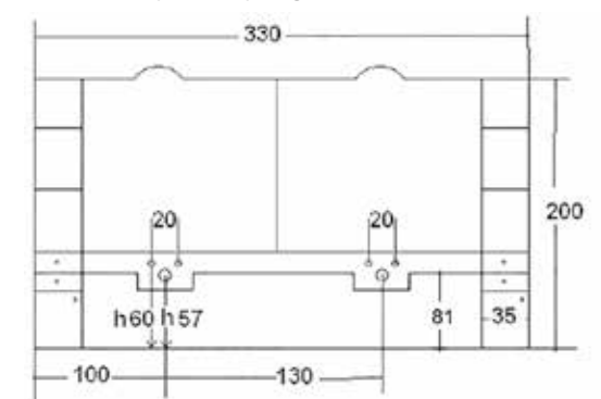
SCHEMA PER LAVELLO TONDO AD INCASSO TECHNICAL DRAWING FOR ROUND BUILT-IN SINK PROFONDITÀ / DEPTH: 45 cm
